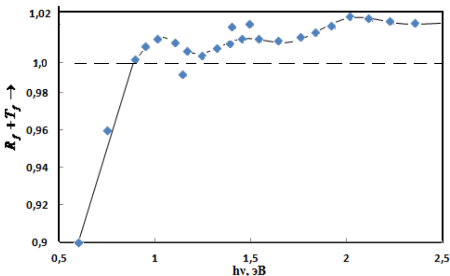
Рис. Спектрофотометрический анализ в пленках сплавов a -Si:H и a -nk-C:H
