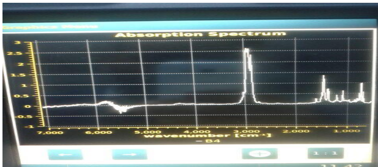
Рис. 2(a,b,c). Облученный бензин АИ-95(В4) при поглощенной дозе ( D=78 кГр) сразу после облучения. с-ZX-440 XL Анализатор жидких топлив использует очень точную почти инфракрасную спектроскопию.
